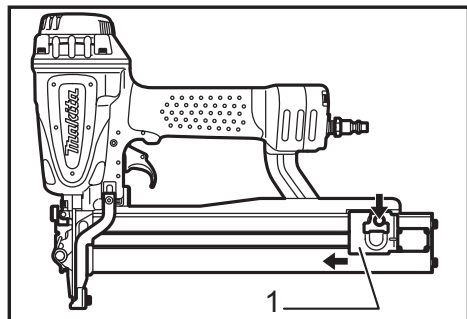
► 1. Pusher
