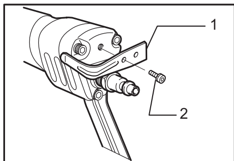
► 1. Gancho 2. Tornillo
